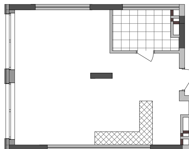
План квартири без перегородок
